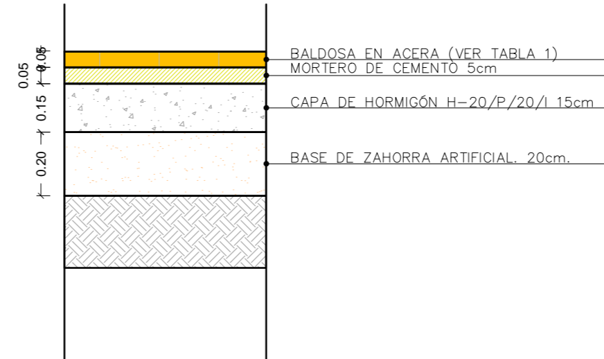
DETALLE BALDOSA EN ACERA SIN ESCALA
