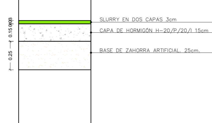
DETALLE CARRIL BICI SIN ESCALA
