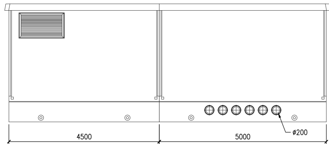
VISTA POSTERIOR
