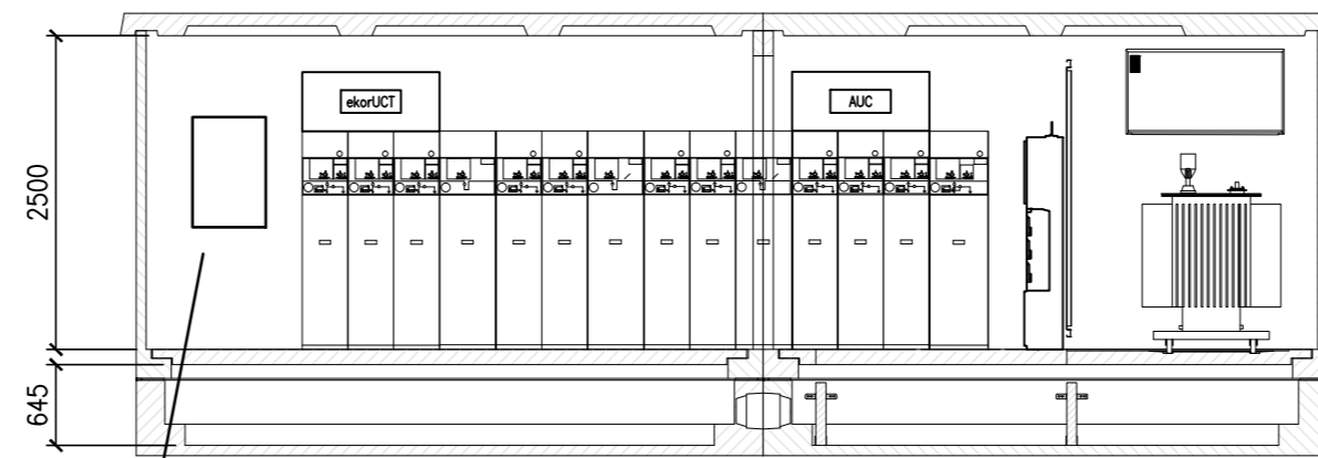
SECCIÓN A-A
