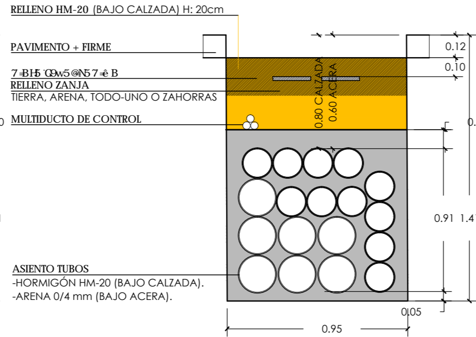
TIPO 6MT+11BT+1R 7Ø200+11Ø160+TRITUBO
