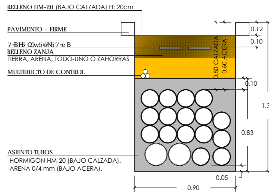
TIPO 1MT+16BT+1R 2Ø200+16Ø160+TRITUBO
