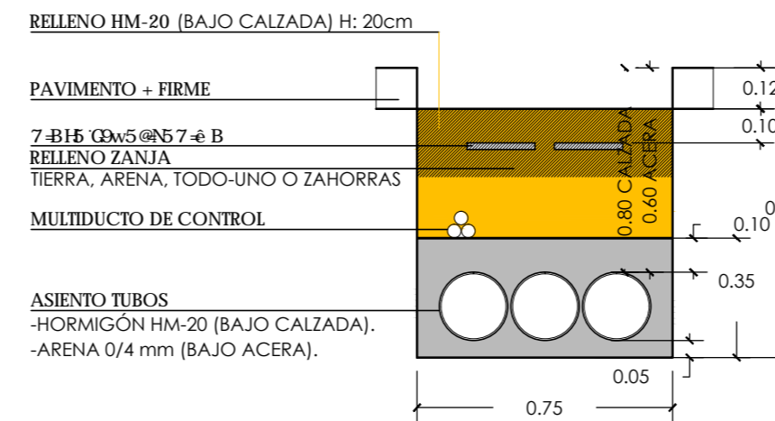
TIPO 2MT+1R 3Ø200+TRITUBO
