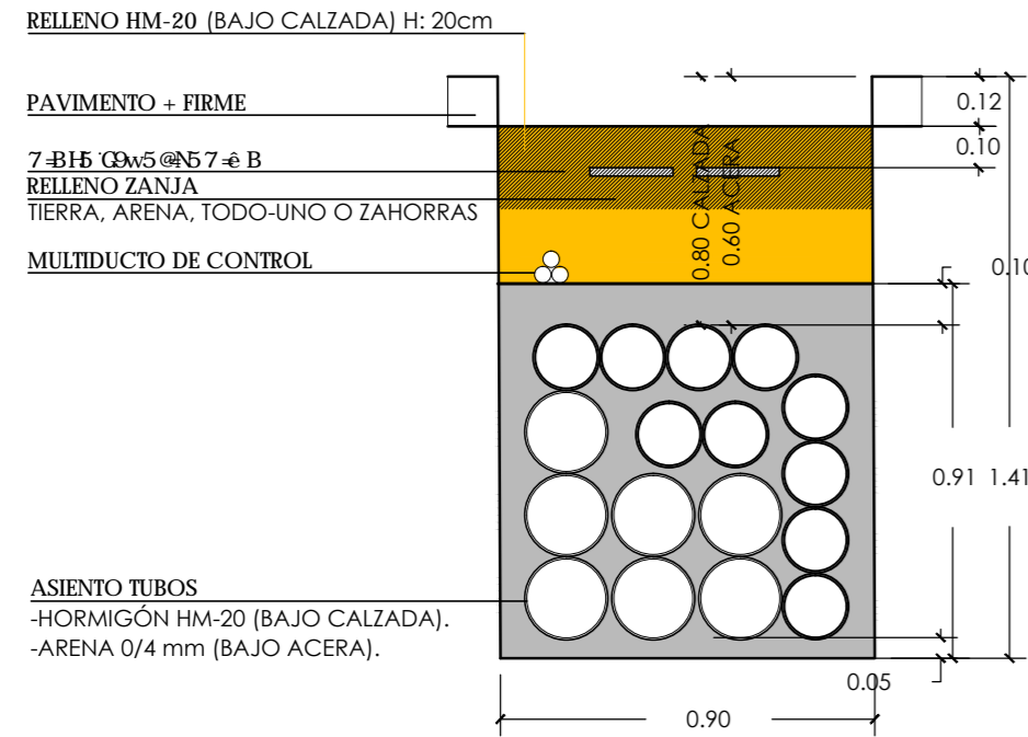
TIPO 6MT+10BT+1R 7Ø200+10Ø160+TRITUBO
