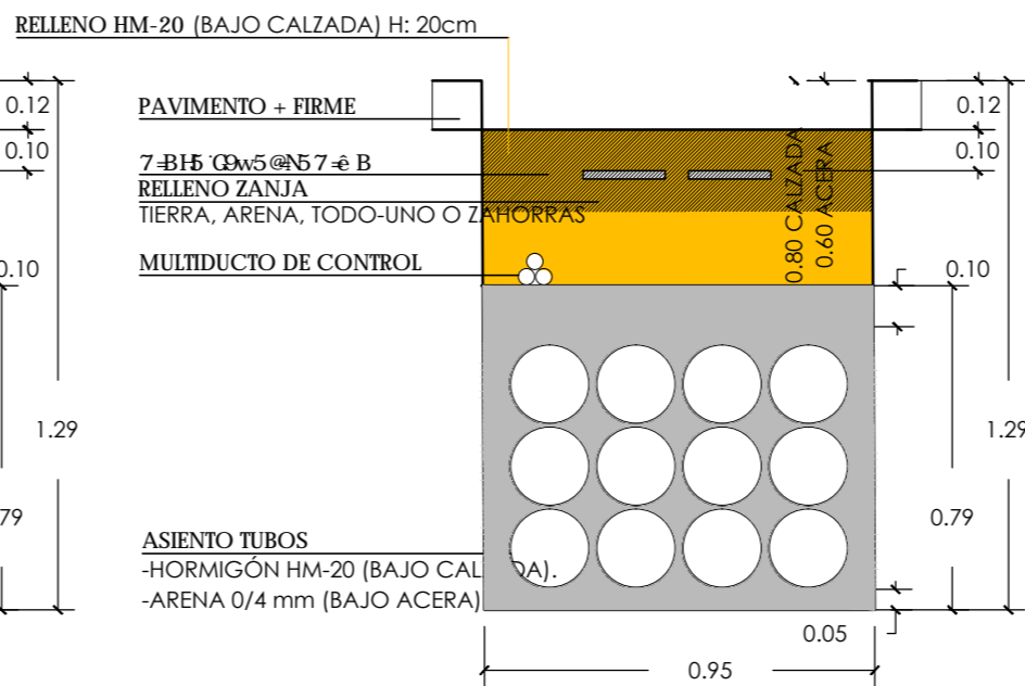
TIPO 11MT+1R 12Ø200+TRITUBO
