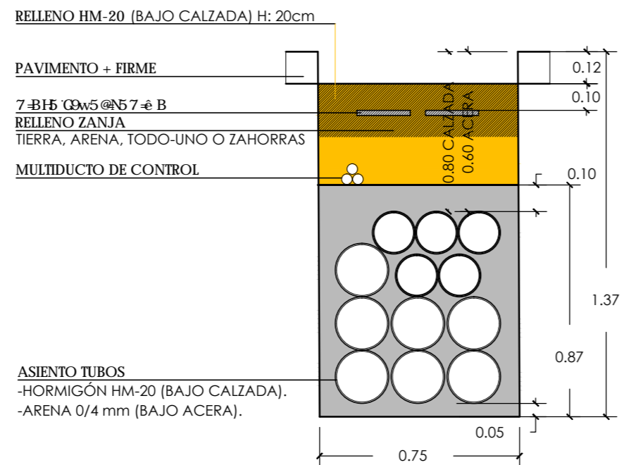
TIPO 6MT+5BT+1R 7Ø200+5Ø160+TRITUBO
