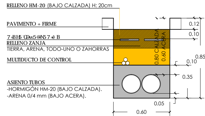
TIPO 1MT+1R 2Ø200+TRITUBO
