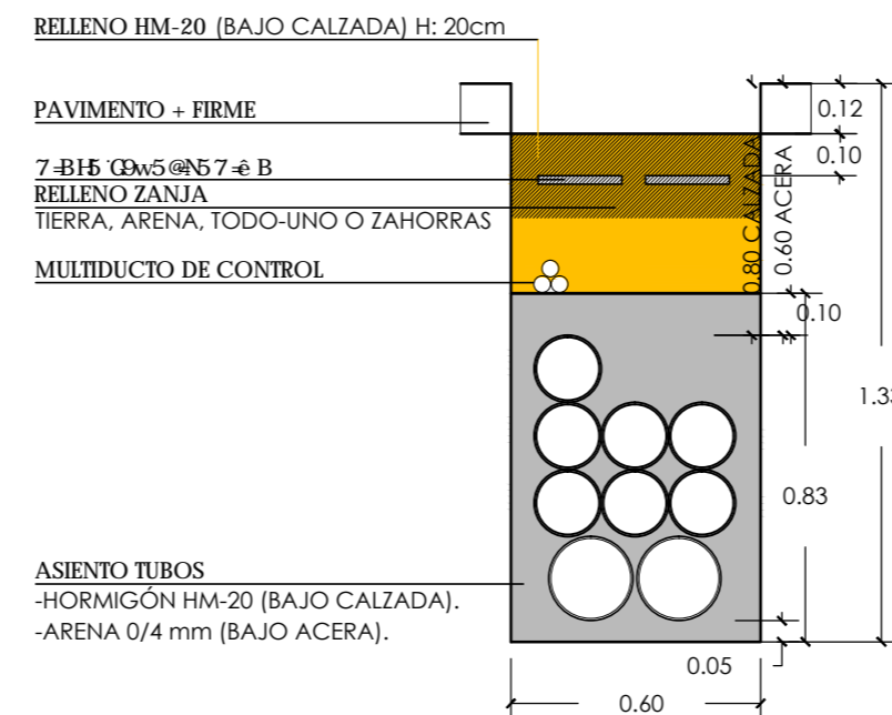
TIPO 1MT+7BT+1R 2Ø200+7Ø160+TRITUBO
