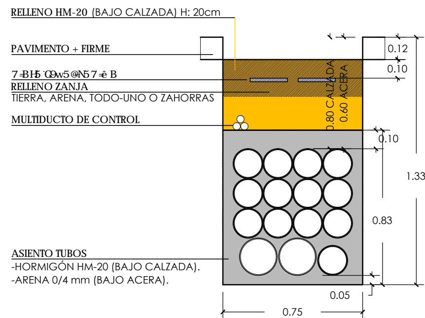
TIPO 1MT+13BT+1R 2Ø200+13Ø160+TRITUBO
