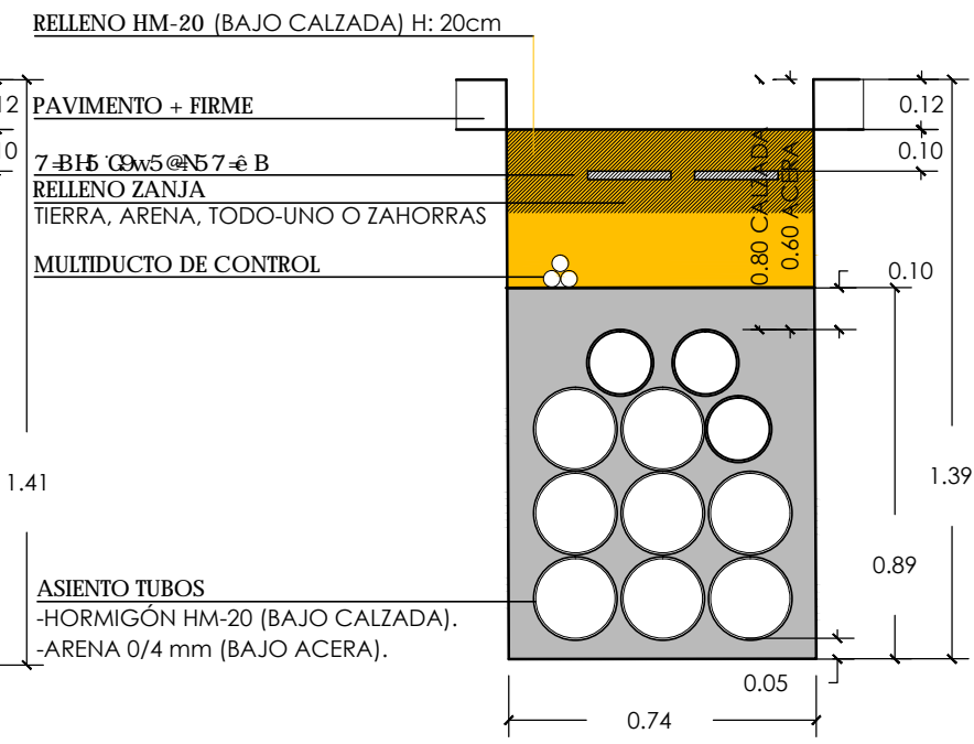
TIPO 7MT+3BT+1R 8Ø200+3Ø160+TRITUBO
