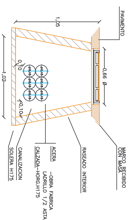
ARQUETAS REGISTRABLES "IN SITU" (TIPO AG) PARA MARCO Y TAPA DE FUNDICION M2/T2 (ACERAS/JARDINES/CALZADAS)
