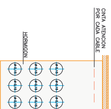
PRISMA N°2 PRISMA 6T DE L.S.B.T. PRISMA 3T DE L.S.M.T.
