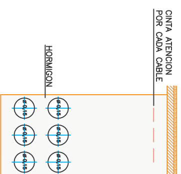
PRISMA N°1 PRISMA 6T DE L.S.M.T.
