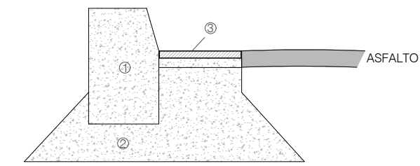
SECCION BORDILLO
