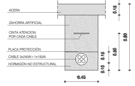
TENDIDO DE UNA LINEA
