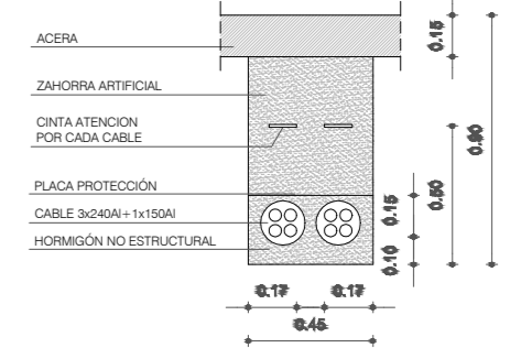
TENDIDO DE DOS LINEAS
