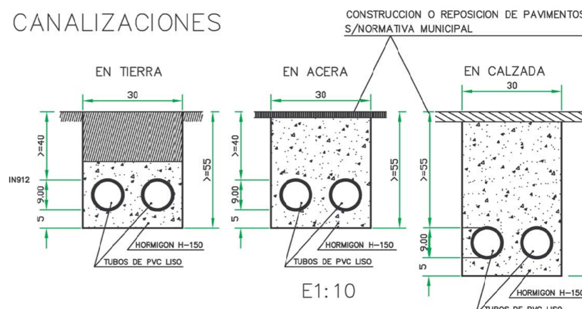
ACOTADO EN CENTIMETROS
