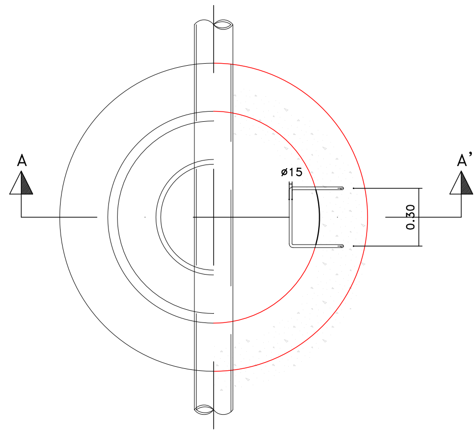
SECCION B-B' POZO DE REGISTRO
